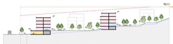
TIPOVÝ REZ OBYTNÉ ULICE
